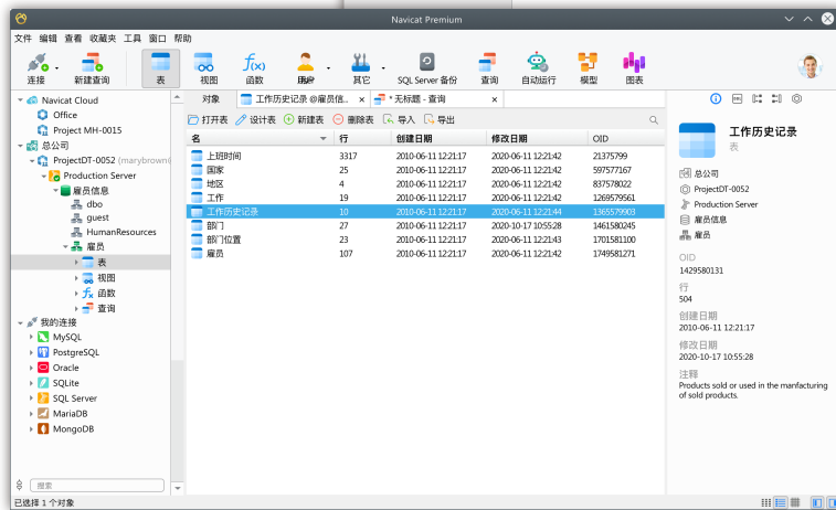
Linux 系统
