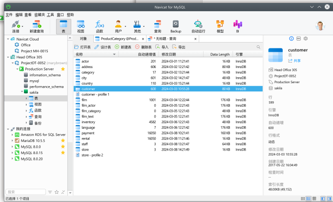
Linux 版本
