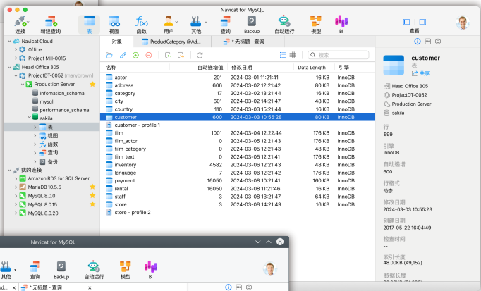
macOS 版本
