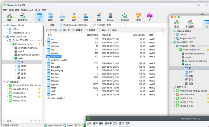
Windows 版本
